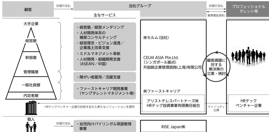
[事業系統図]
